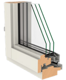
Genomskäring
