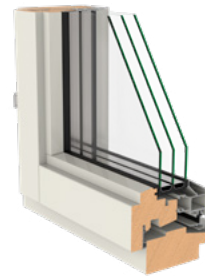
Genomskärning
