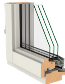
Genomskärning
