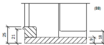
Ventilerad tröskel
