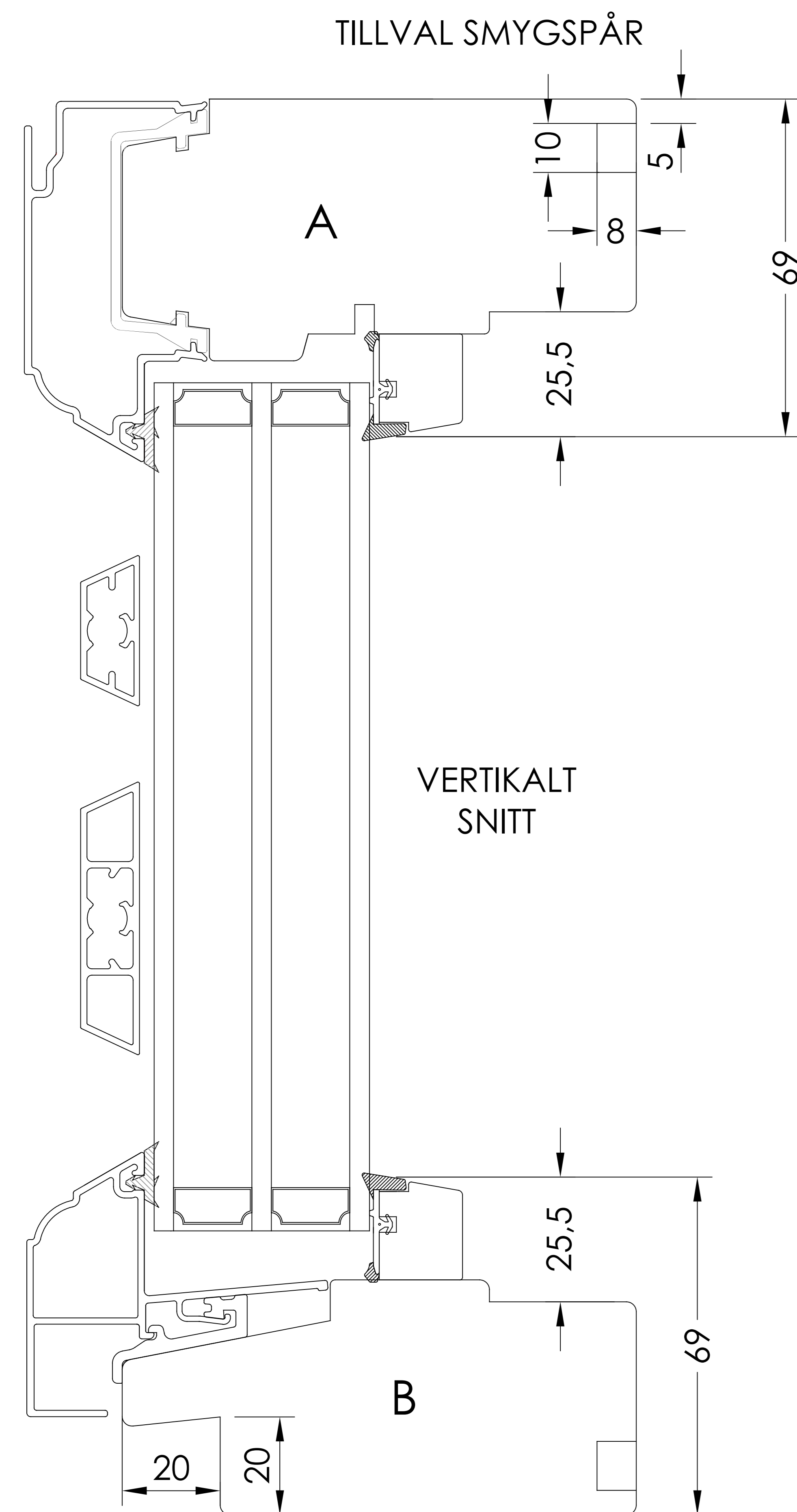
VERTIKALT SNITT TILLVAL - Norgenäsa
