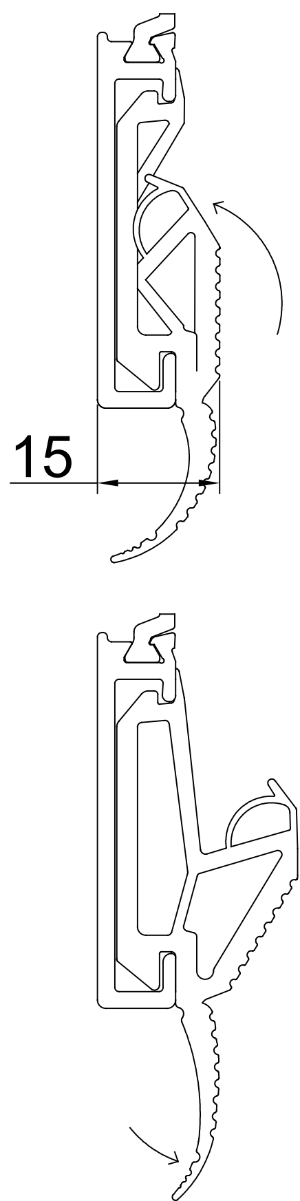
- Flexing EPDM-rubber
